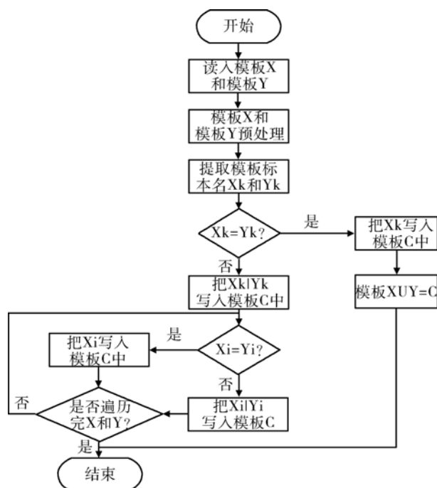
图3 模式泛化路径
