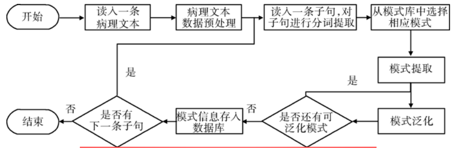
图 1 结构化信息抽取系统流程
