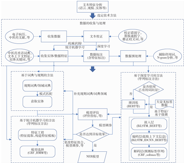
图 3 NER 实现路线
