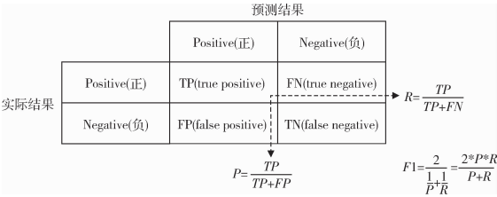
图 2 评价指标计算公式
